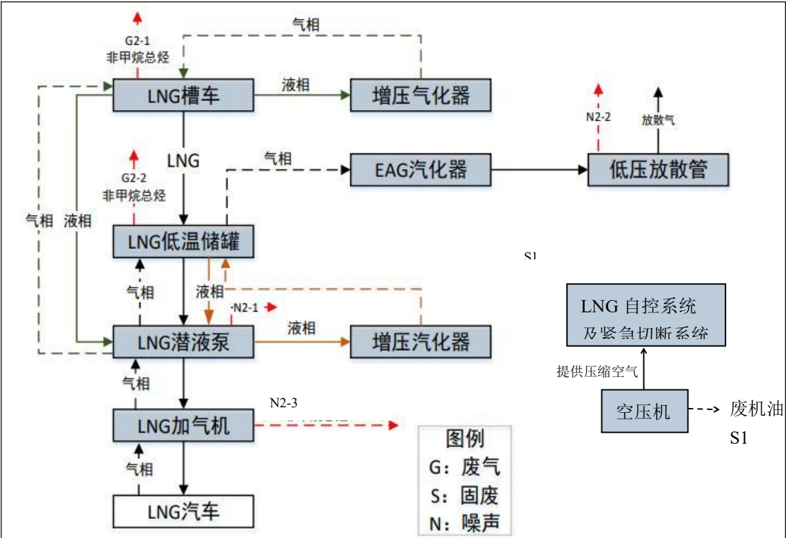
图 2-1 LNG 泄气、加气流程图
